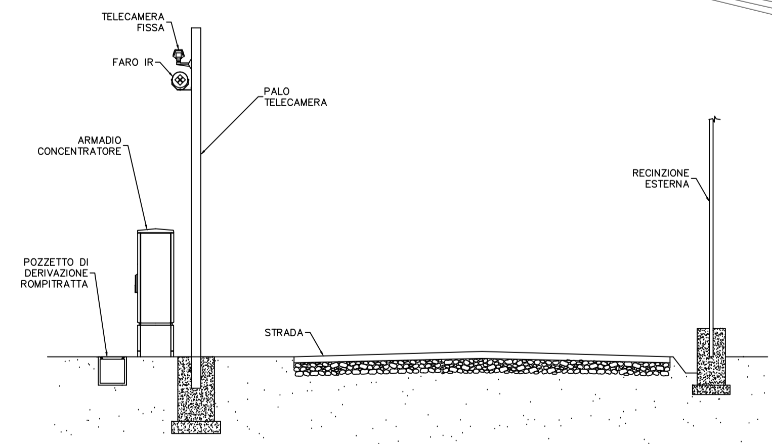
SEZIONE LATERALE
