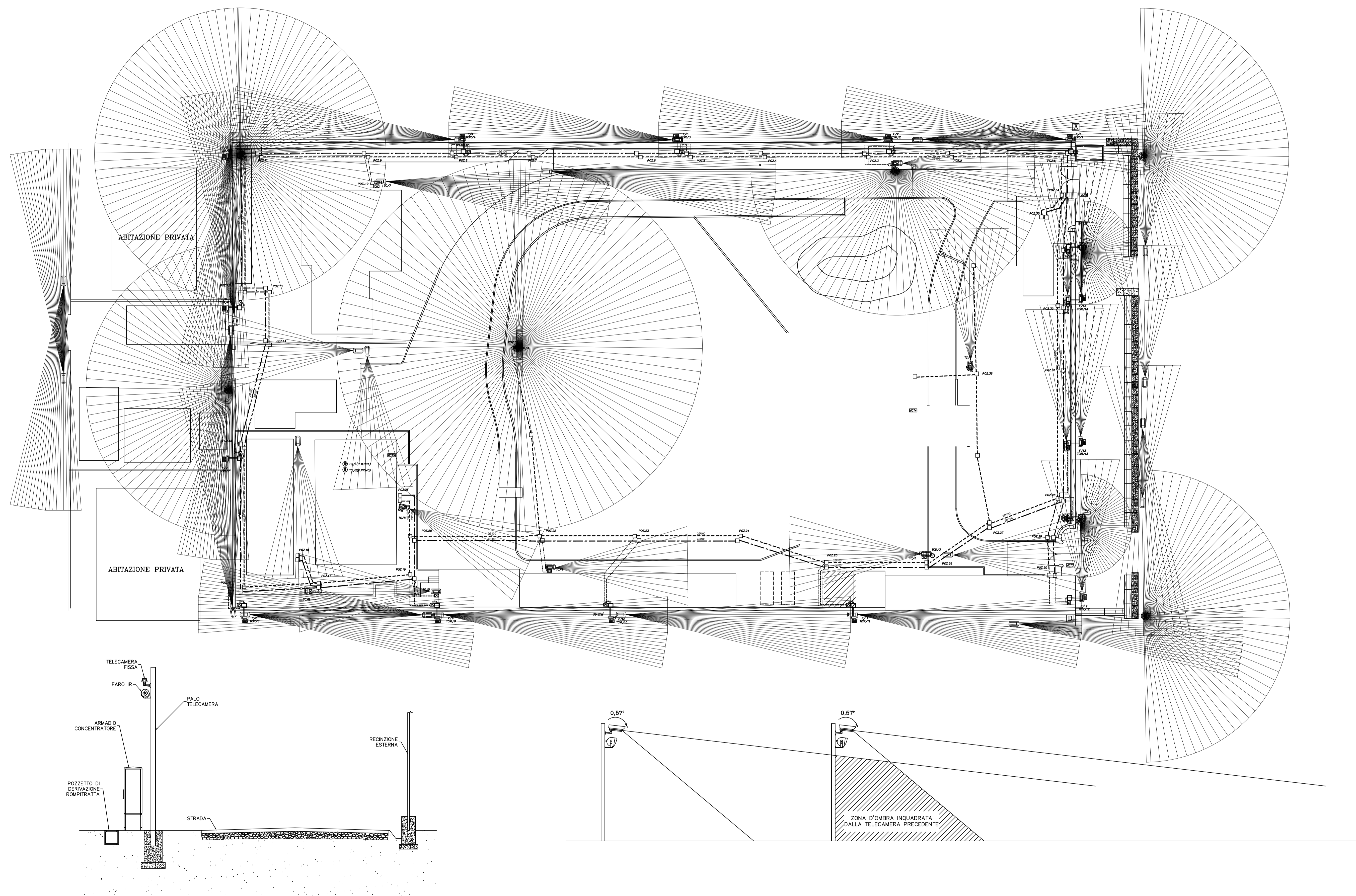
COPERTURA TELECAMERA FISSA ANGOLO PIANO VERTICALE 12° INCLINAZIONE 0,57°
